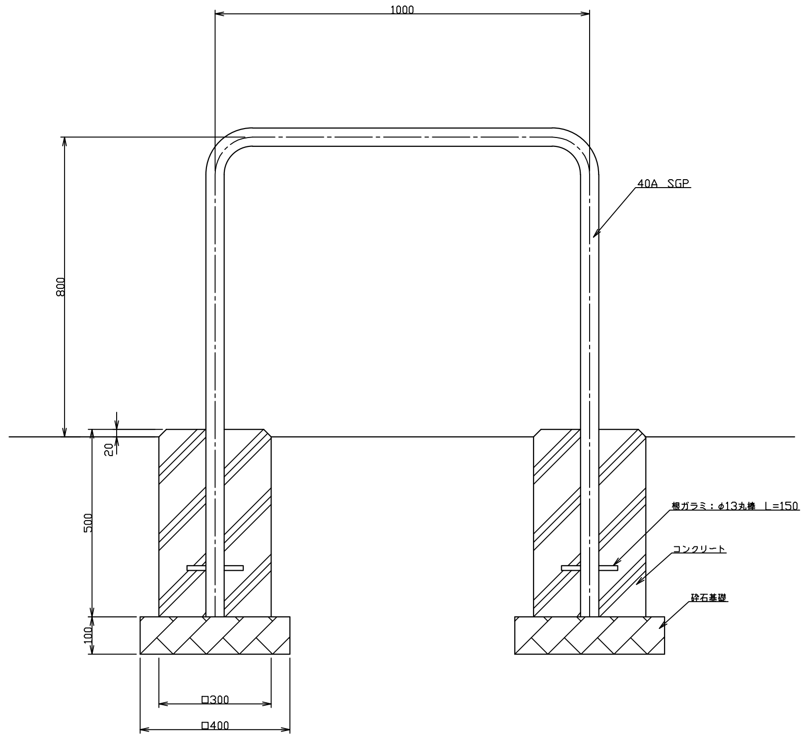
正面図 S=1:10
