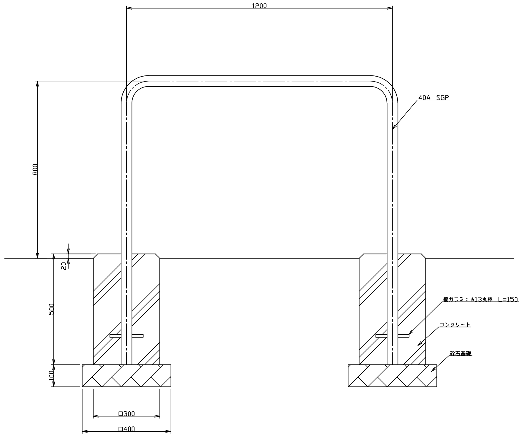
正面図 S=1:10
