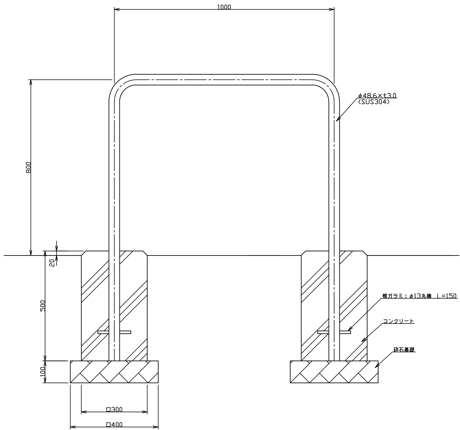
正面図 S=1:10
