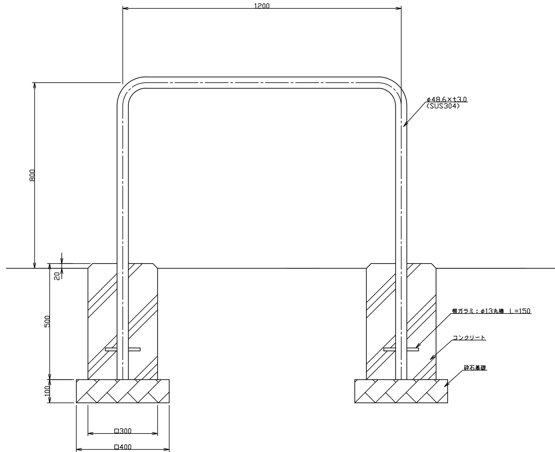
正面図 S=1:10
