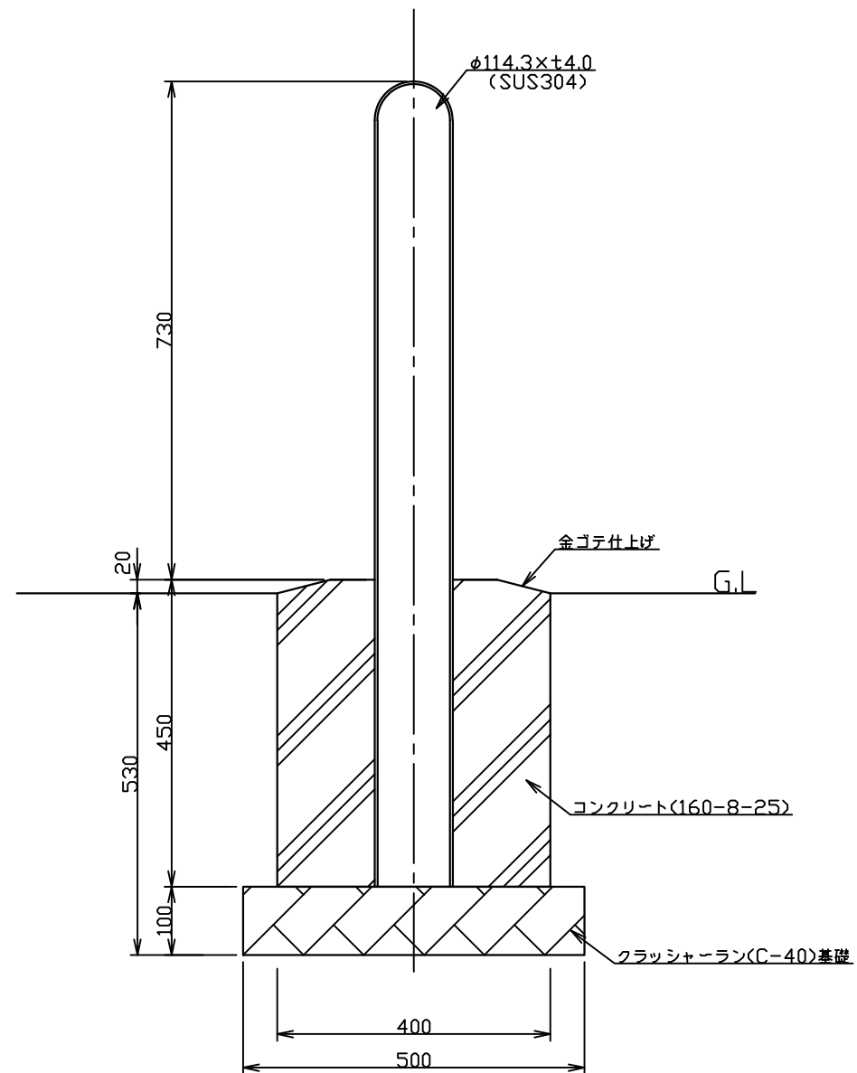
正面図 S=1:10
