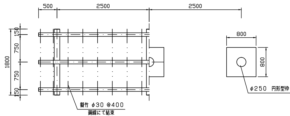
平面及び基礎伏図 S=1:50
