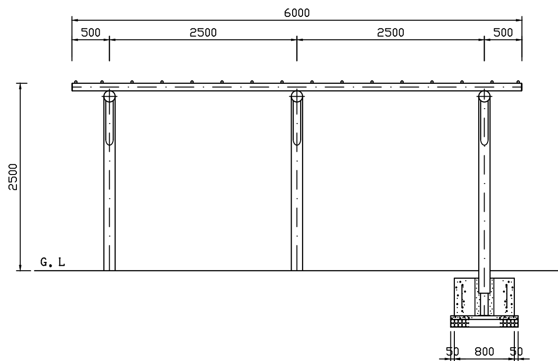
立面図 S=1:50
