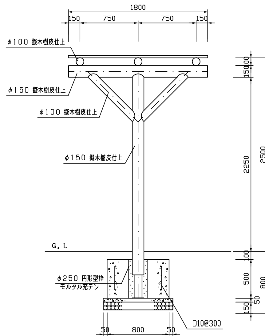
側面図 S=1:30
