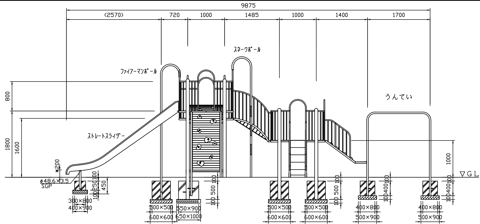
A視立面図 S=1:50
