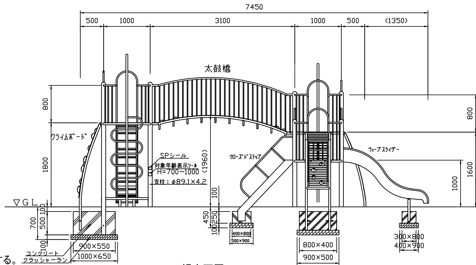
B視立面図 S=1:50
