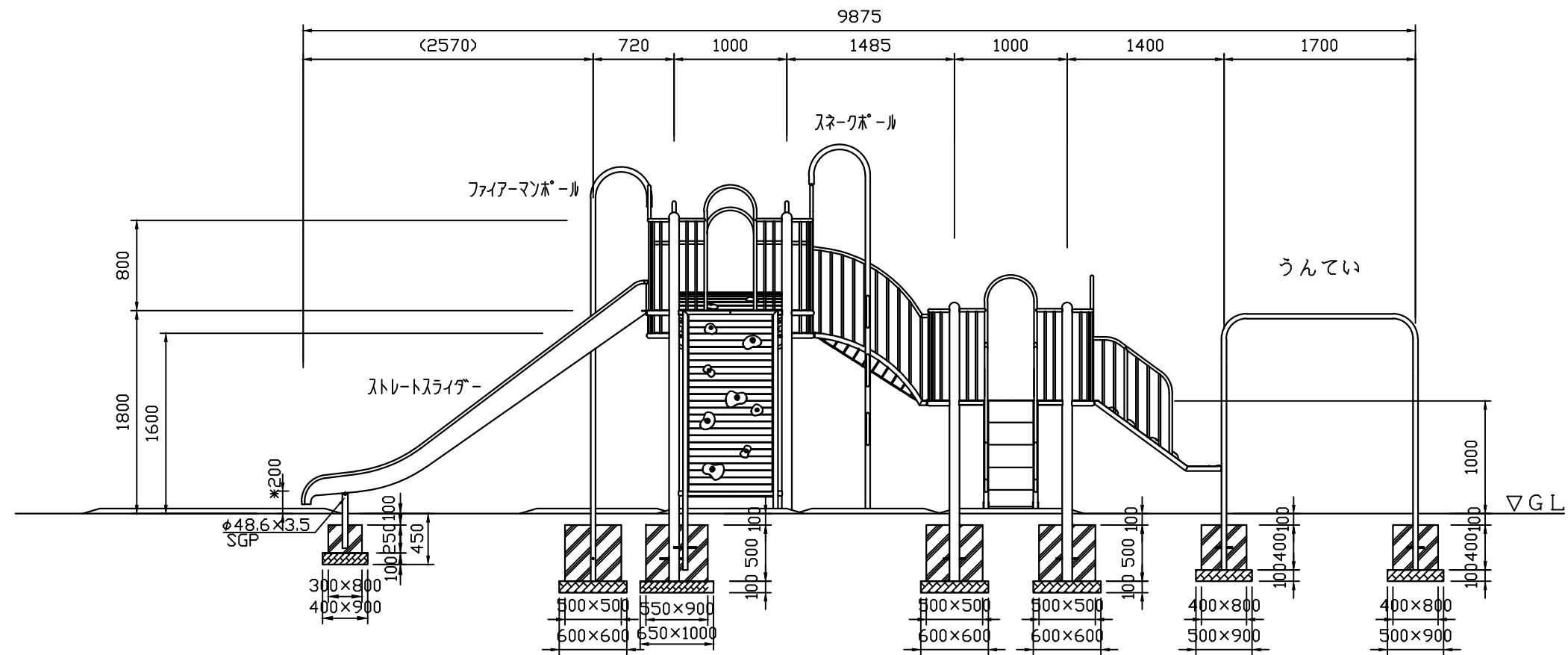
A視立面図 S=1:50
