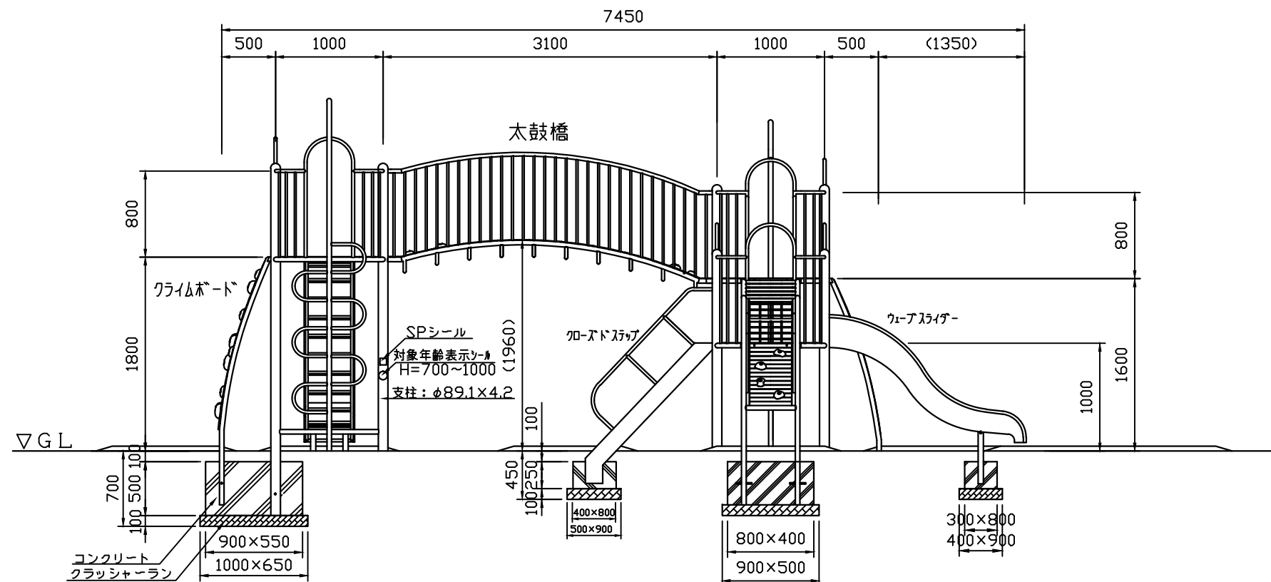
B視立面図 S=1:50
