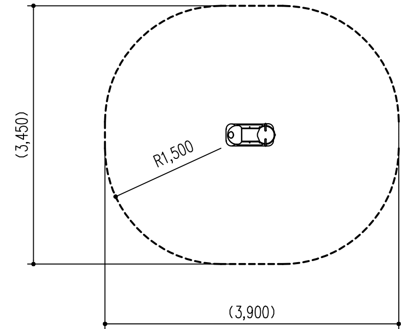
安全領域平面図 S=1:50
