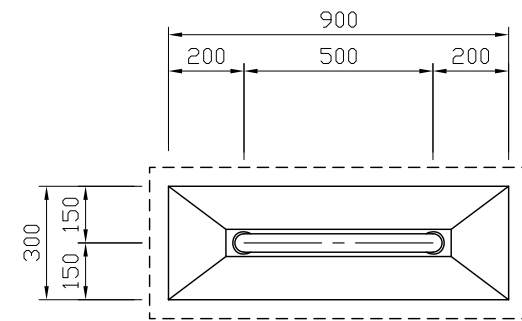
平面図 S=1:20
