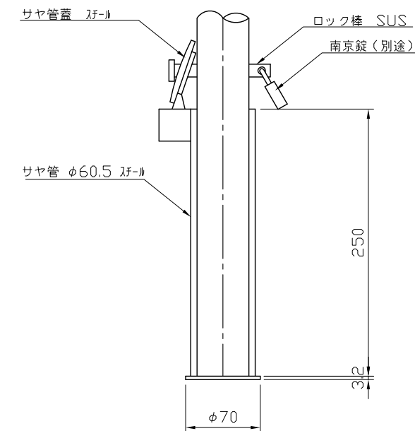
サヤ管詳細図 S=1:5
