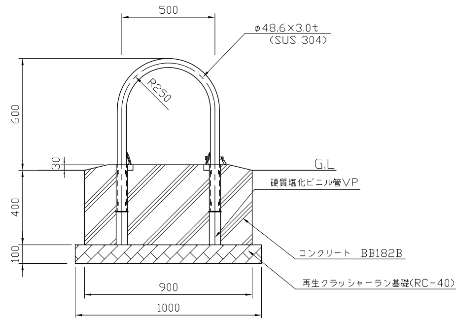
立面図 S=1:20
