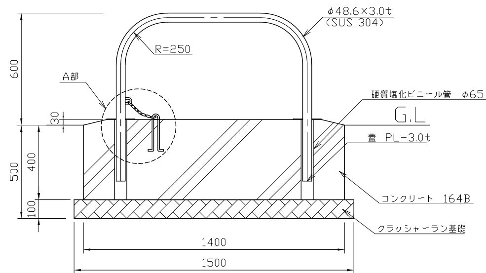
立面図 S=1:20
