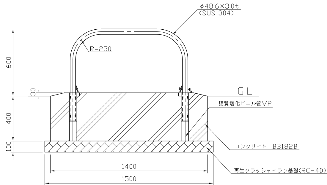
立面図 S=1:20
