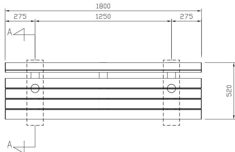
平面図 S=1:20
