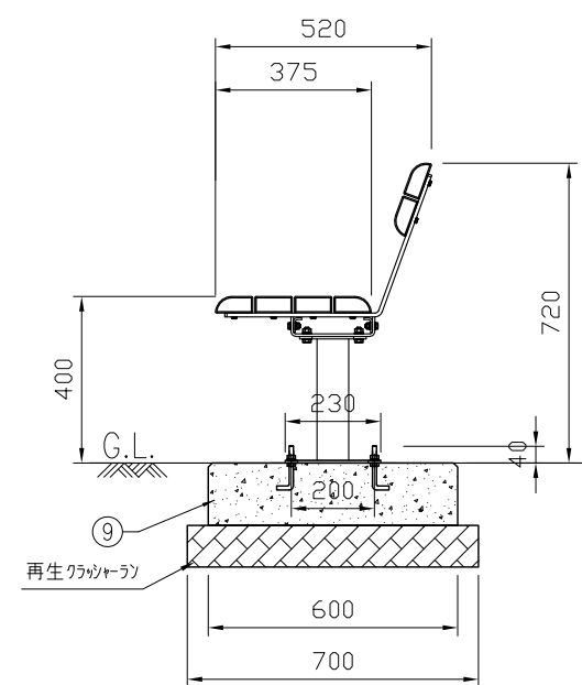
側面図 S=1:20
