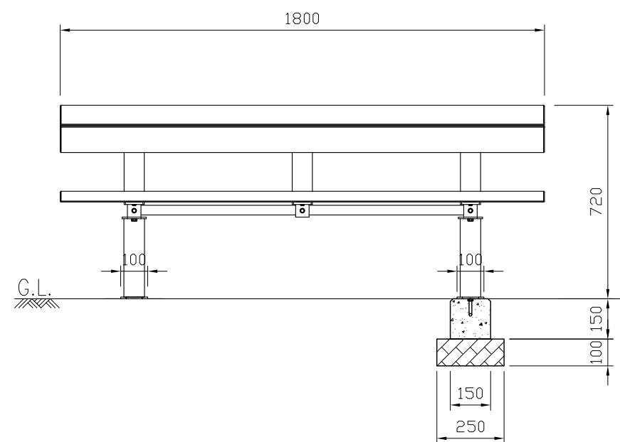
正面図 S=1:20
