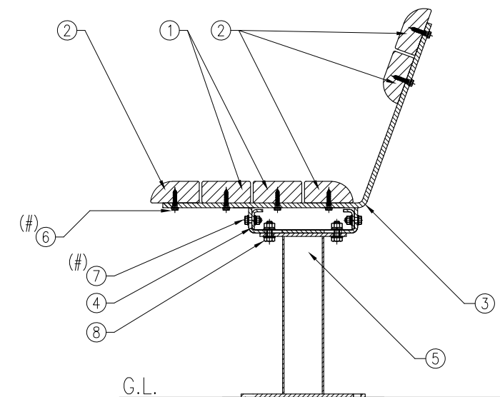
組付断面図(A-A矢視図) S=1:10
