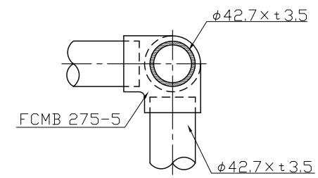
B部詳細図 S=1:5
