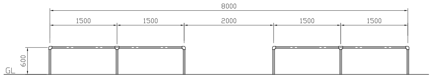
側面図 S=1:50
