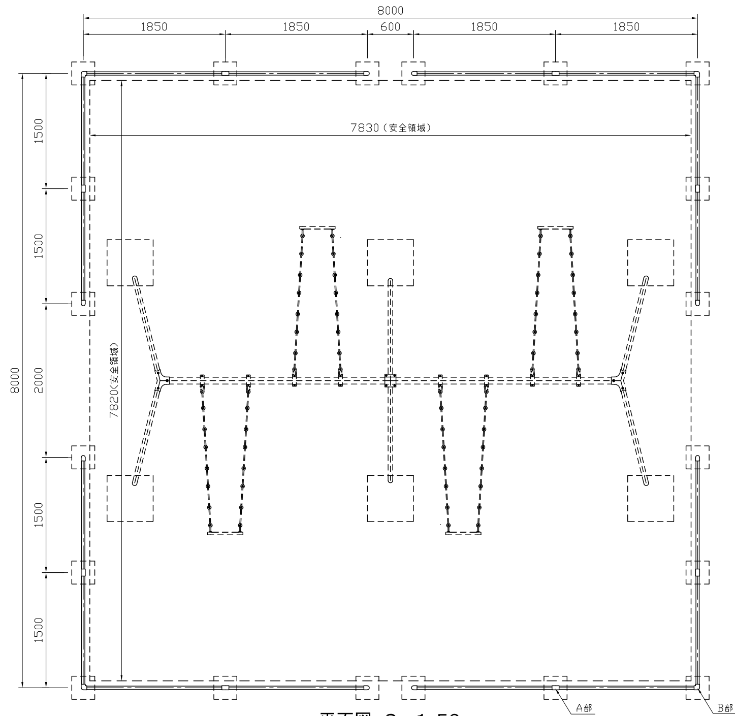
平面図 S=1:50
