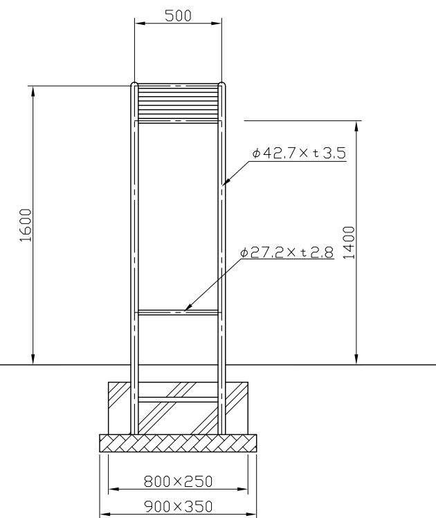
側面図 S=1:30
