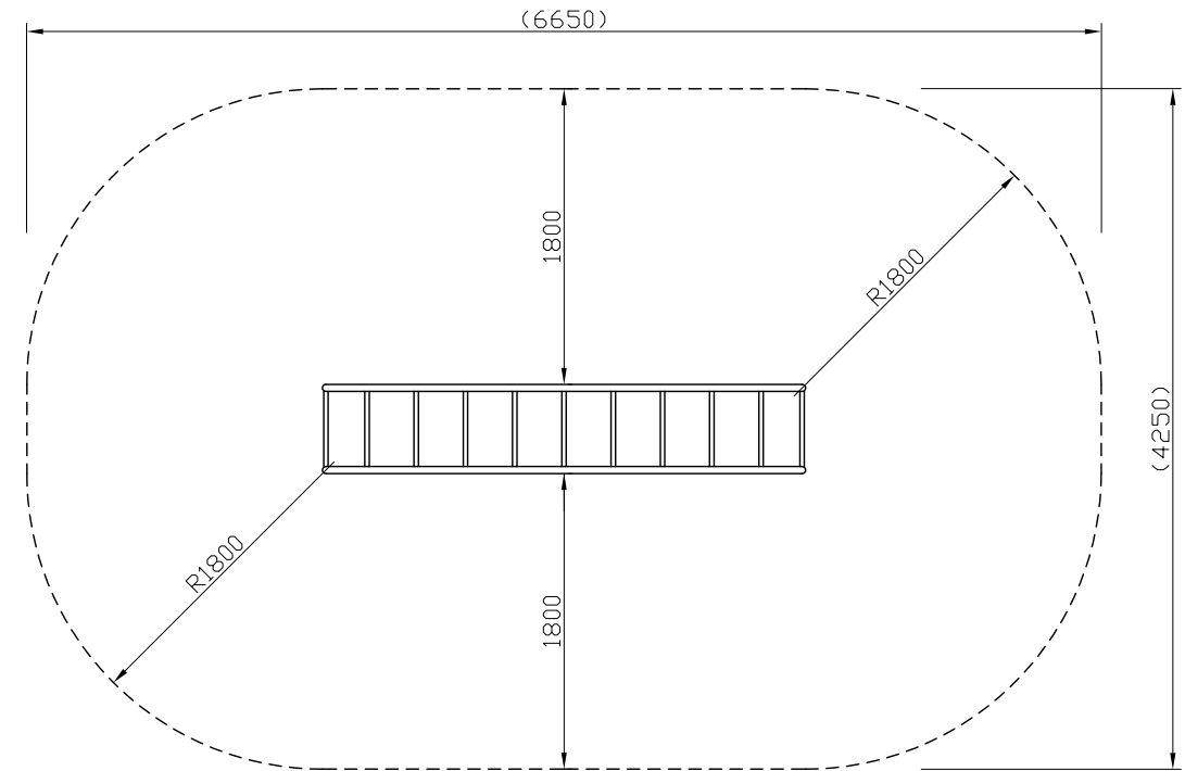
安全領域平面図 S=1:50
