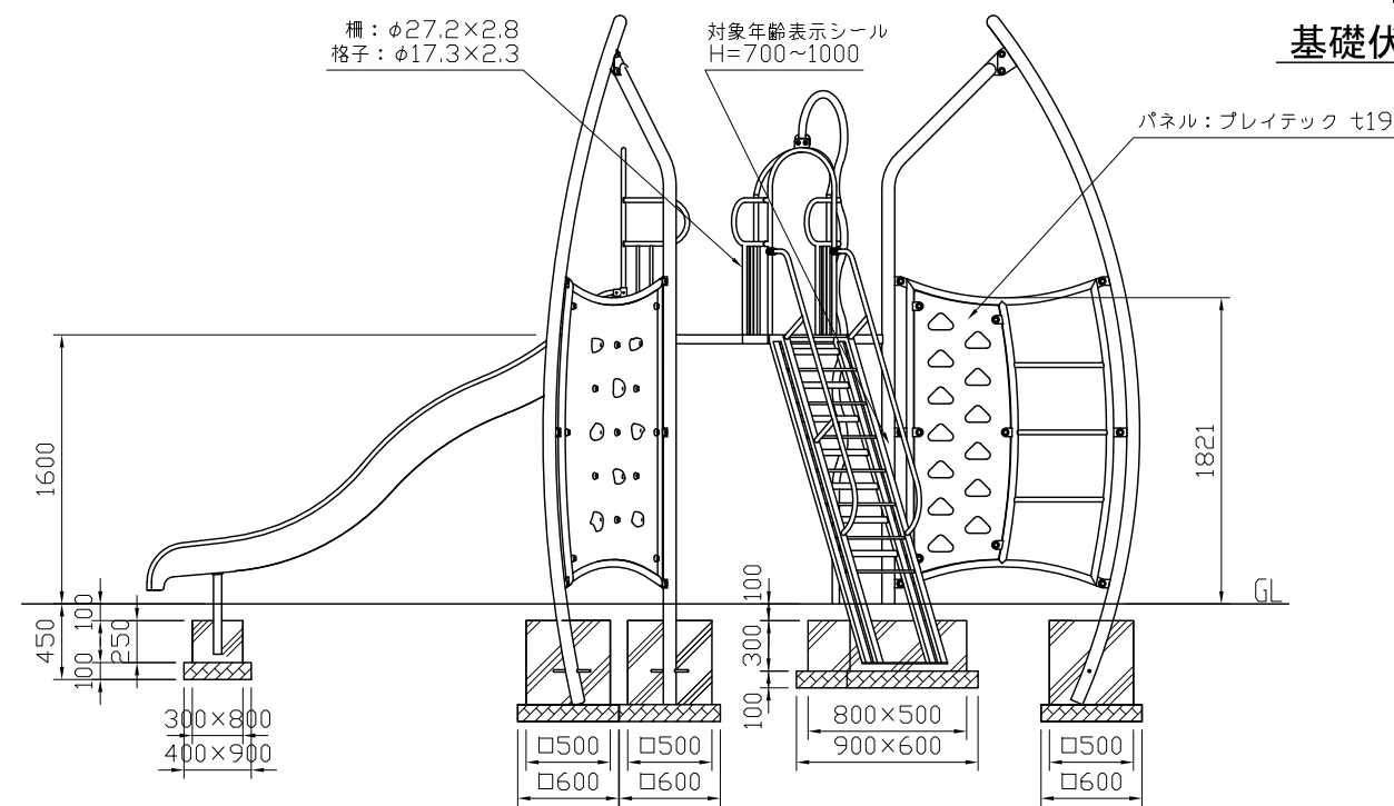
側面図 S=1:50
