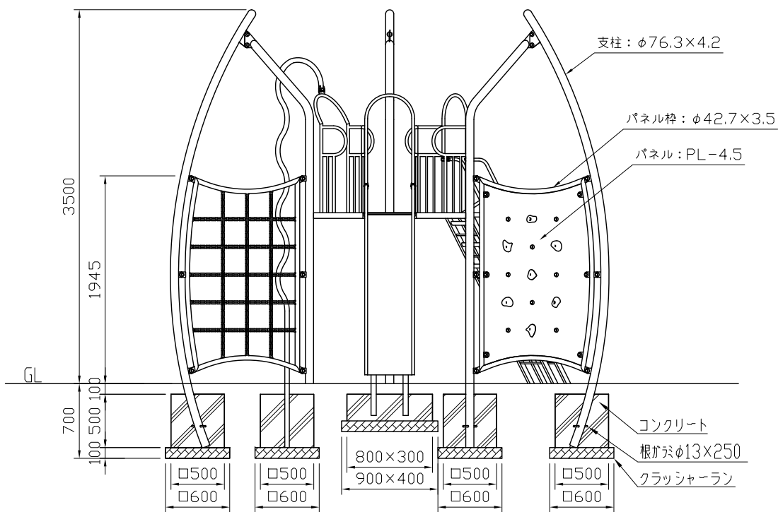
正面図 S=1:50
