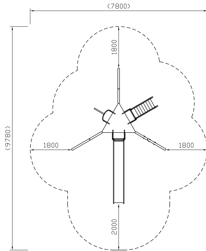
安全領域平面図 S=1:100
