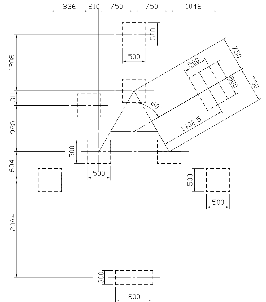
基礎伏図 S=1:50
