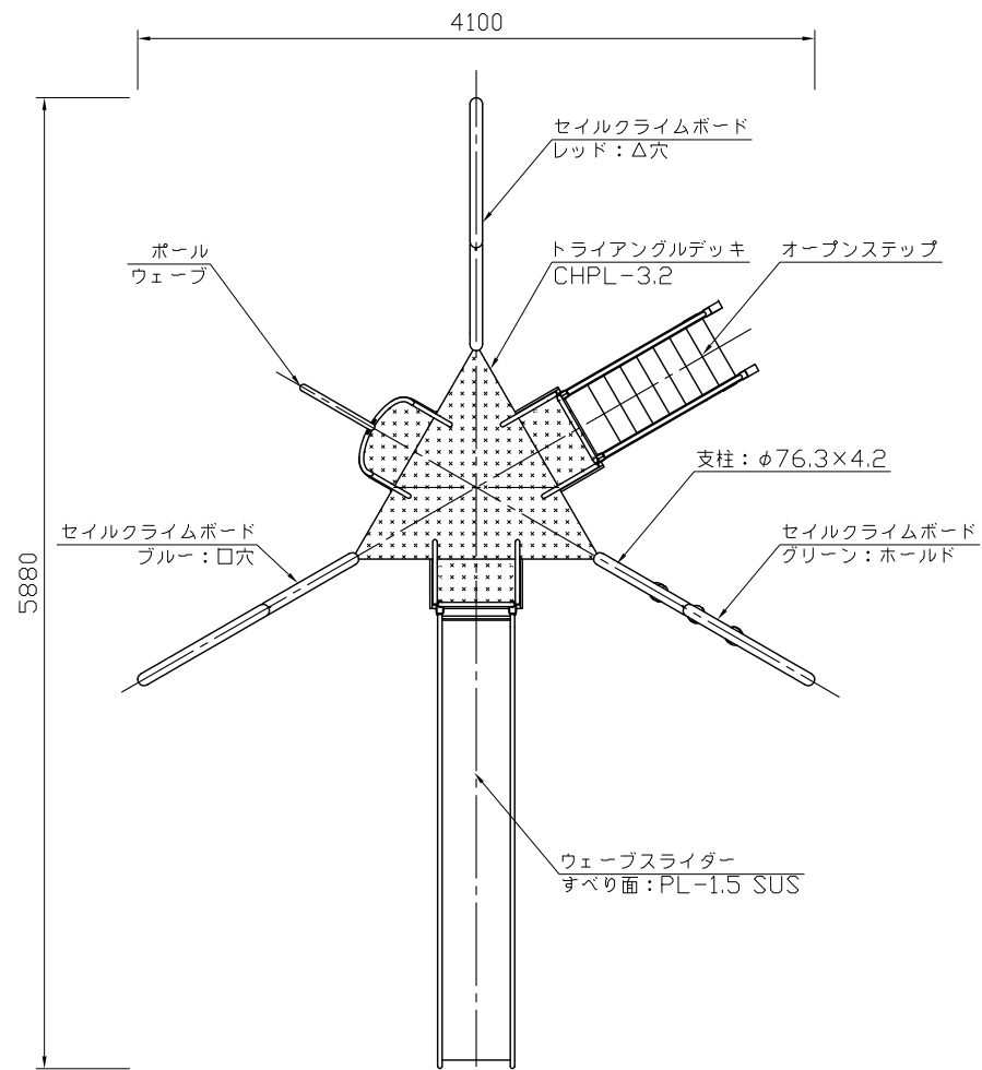
平面図 S=1:50
