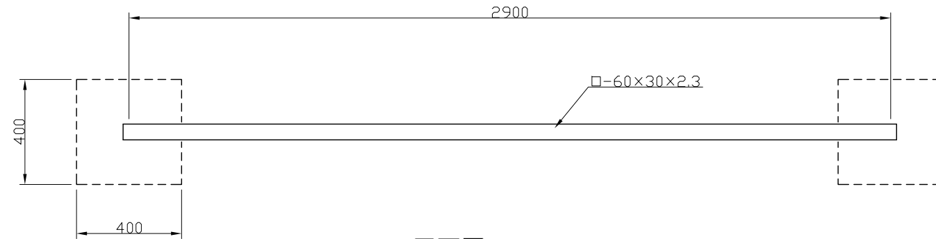
平面図 S=1:20
