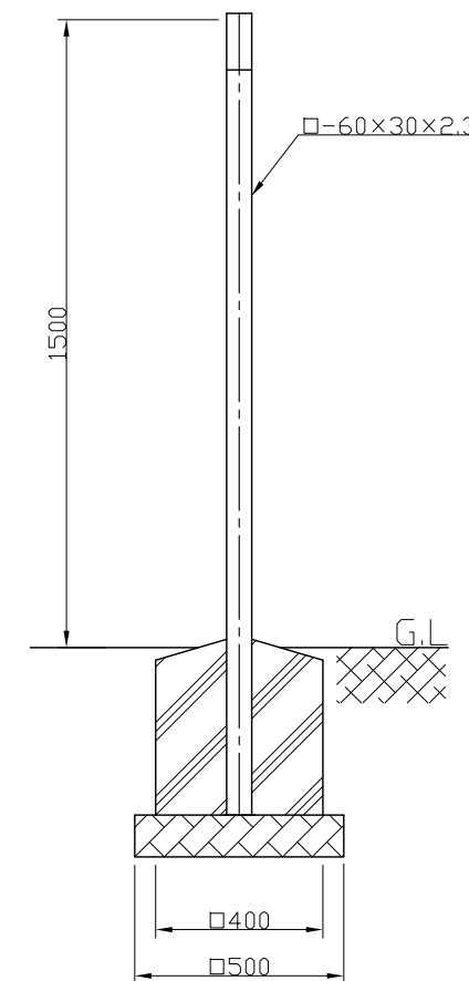
側面図 S=1:20
