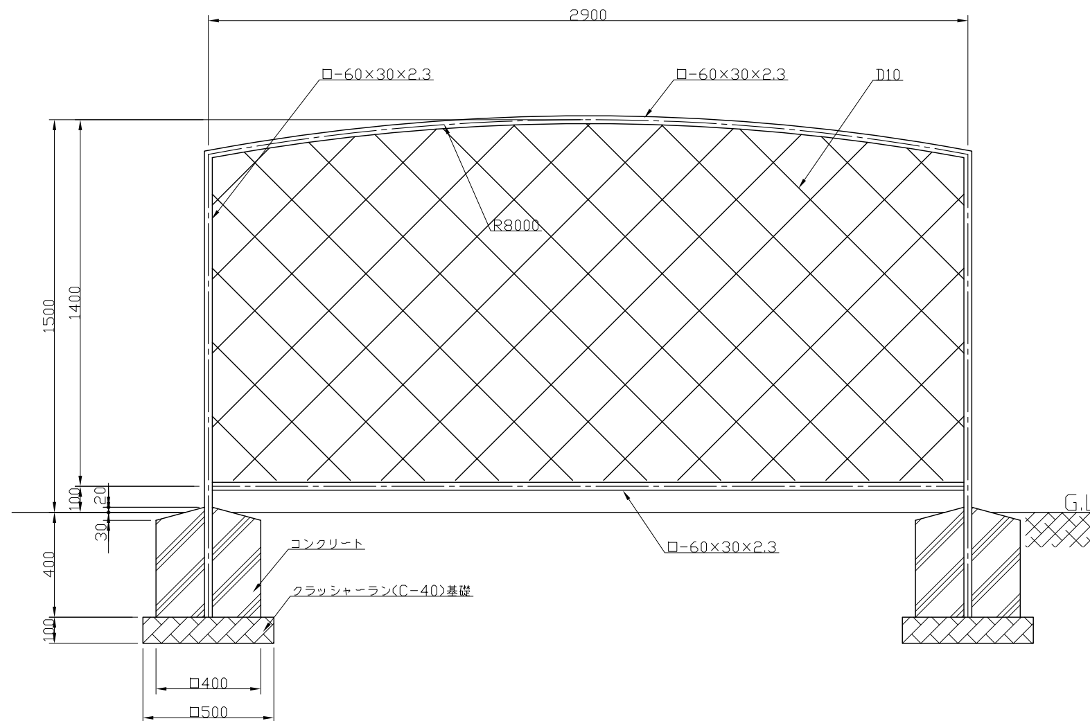
正面図 S=1:20
