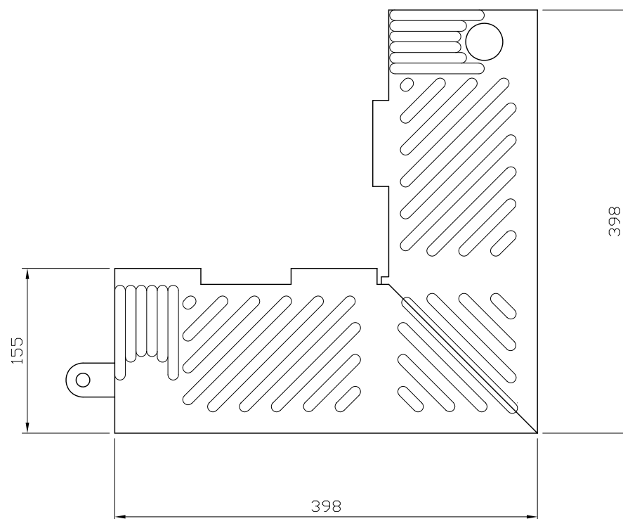
TSX455 スロープエッジコーナ
