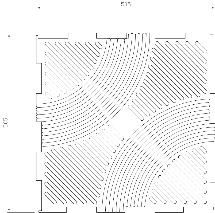
平面図 S=1:5
