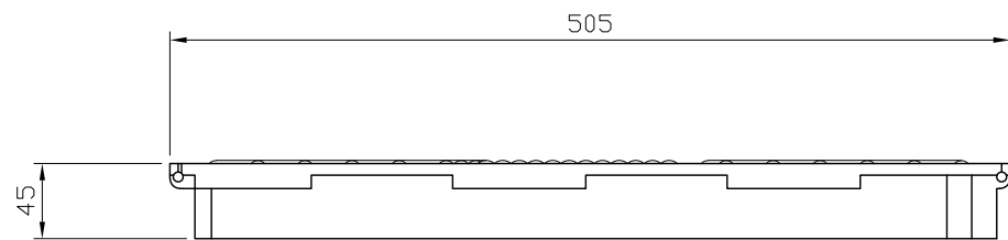
側面図 S=1:5
